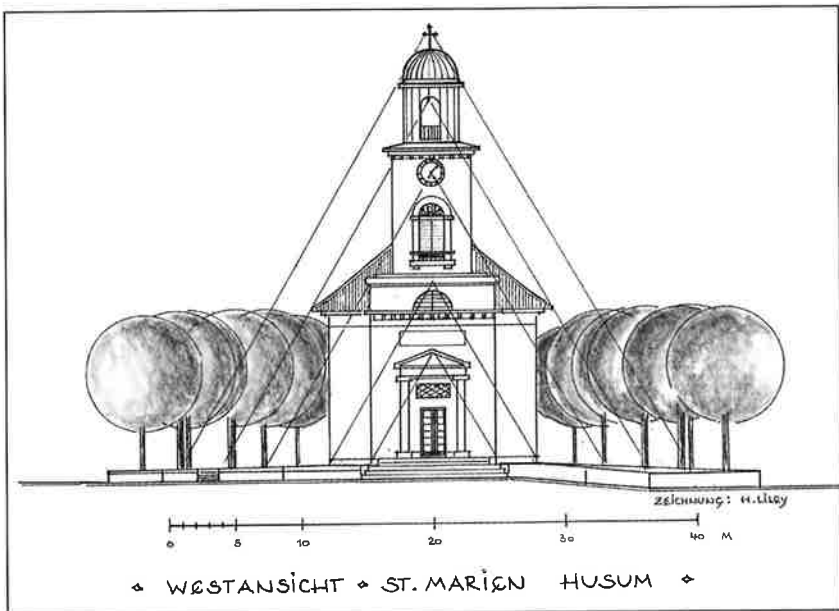
Abb. 4: Ansicht von Westen, Idealschema. Zeichnung von Helmut Liley
