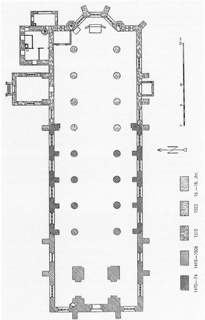
Abb. 1: Horst Appuhn (1953): Rekonstruierter Grundriß der Alten St.-Marien-Kirche Husum
