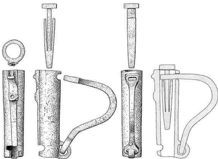
Abb. 7: Vorhängeschloß. M 1:2
